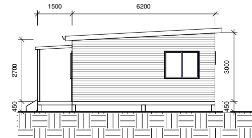
5 Side2 Elevation 1 : 100
