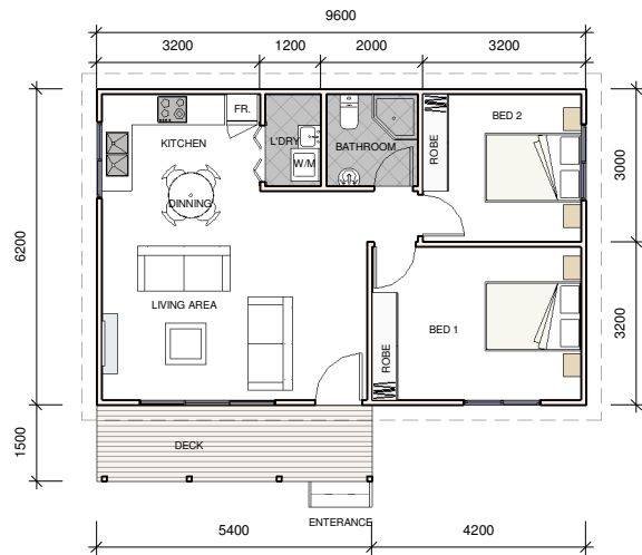
1 Floor Plan 1 : 100
